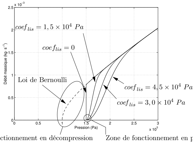
FIG. 4.5 – Fonctionnement des dispositifs de sortie et influence du coefficient correcteur sur le débit massique de sortie
