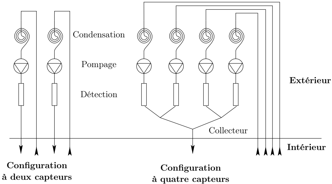
FIG. 3.14 – Les configurations possibles d'utilisation des capteurs à fibre optique dans l'autocuiseur
