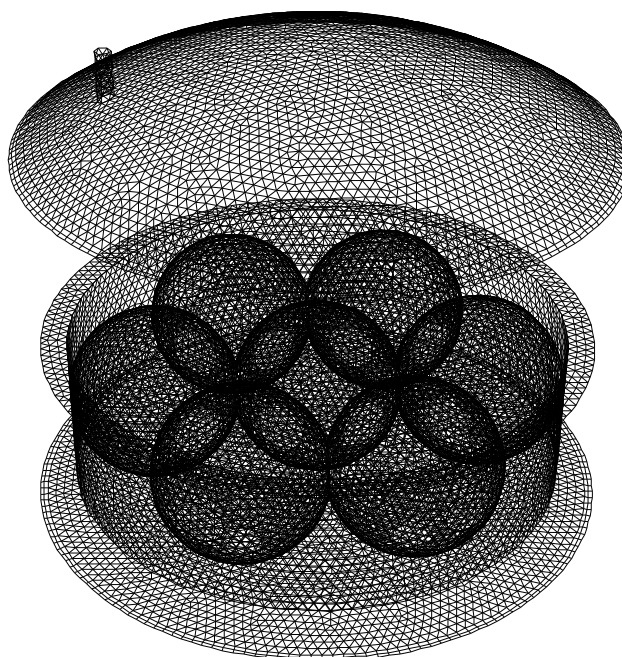
FIG. 4.17 – L'autocuiseur maillé
