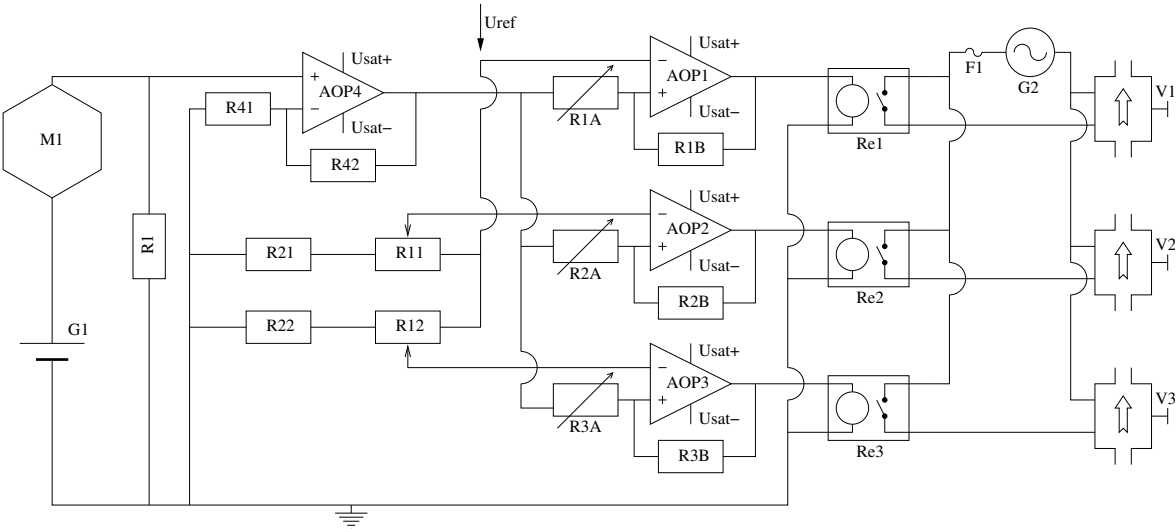
FIG. 7.6 – Montage de régulation de pression par sortie des gaz
