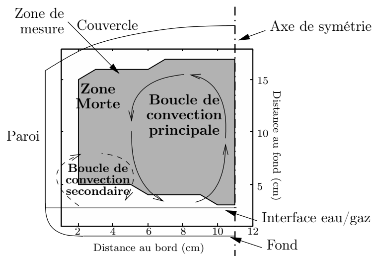
FIG. 5.4 – Interprétation des cellules de convection
