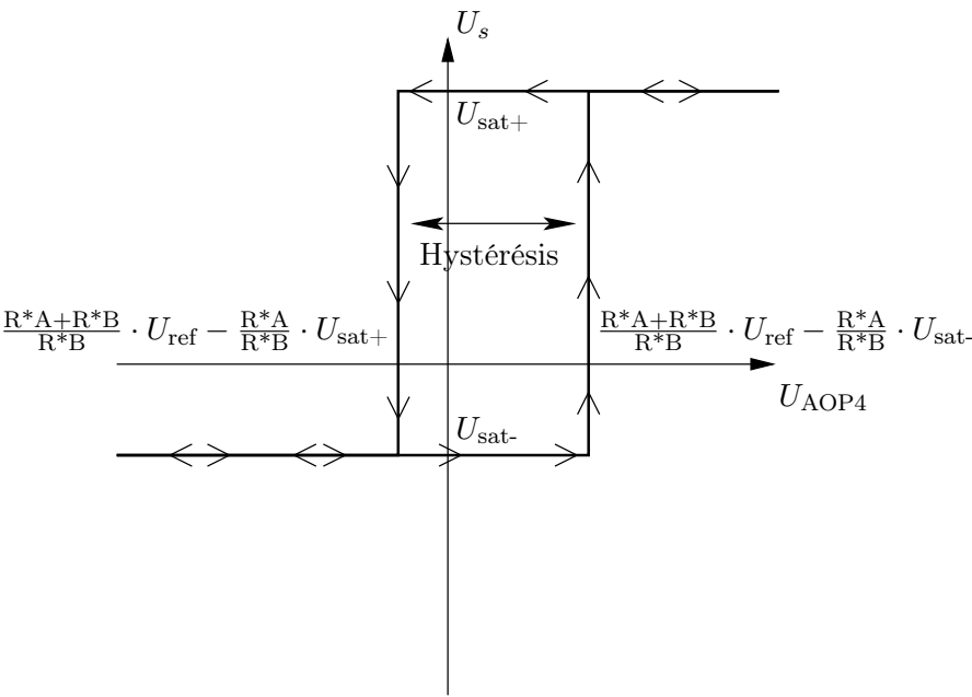
FIG. 7.7 – Caractéristique générale électrique du montage trigger
