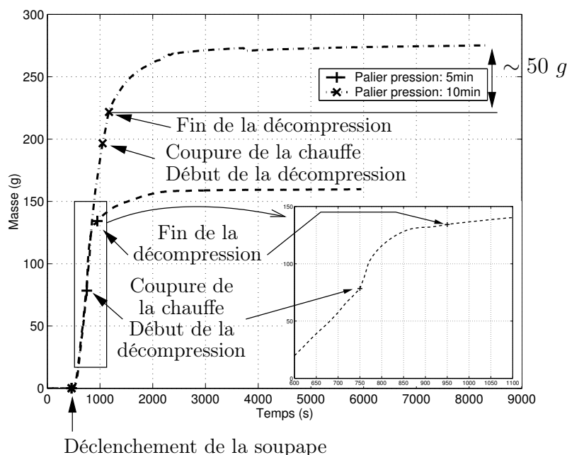
FIG. 3.13 – L'évolution de la masse d'eau récupérée
