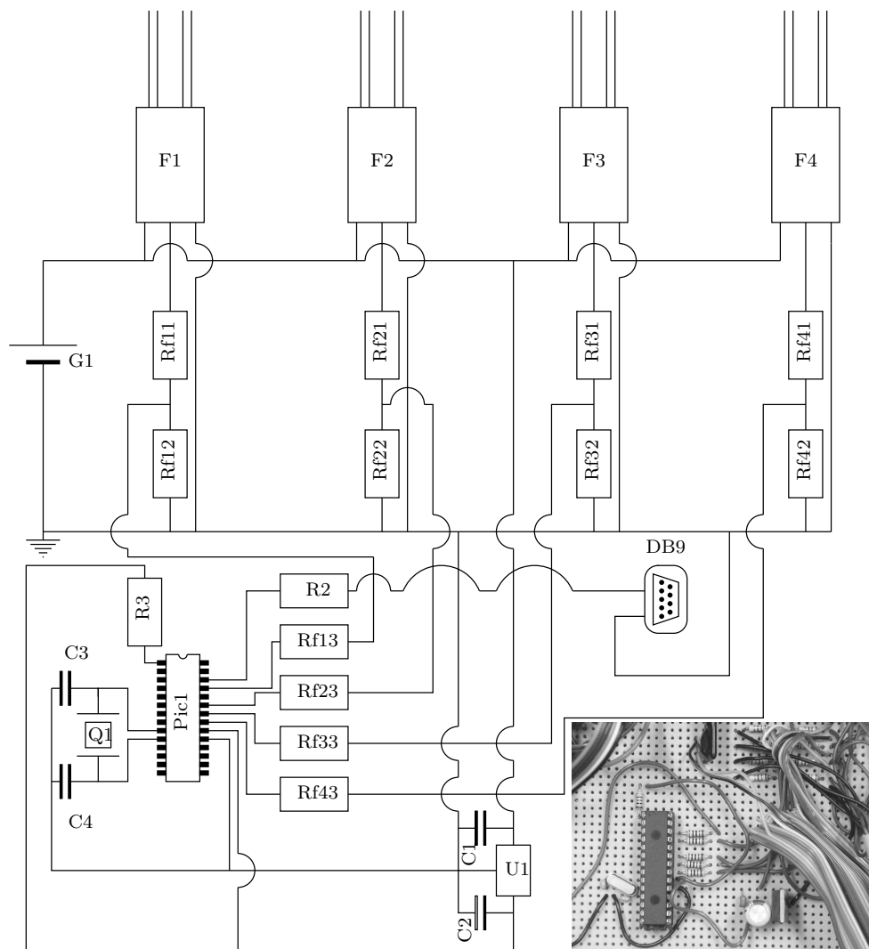
FIG. 7.5 – Schéma électrique de montage des capteurs à fibre optique
