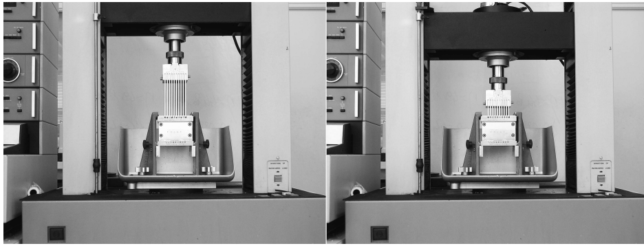
FIG. 3.27 – La course complète de la traverse dans la cellule de Kramer
