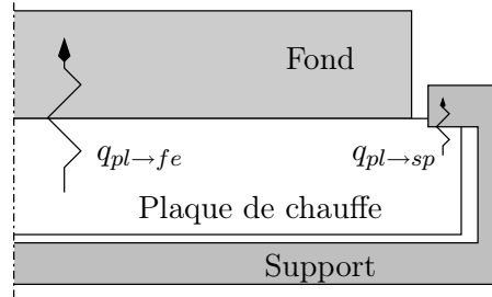
FIG. 4.8 – Schéma des flux de contact
