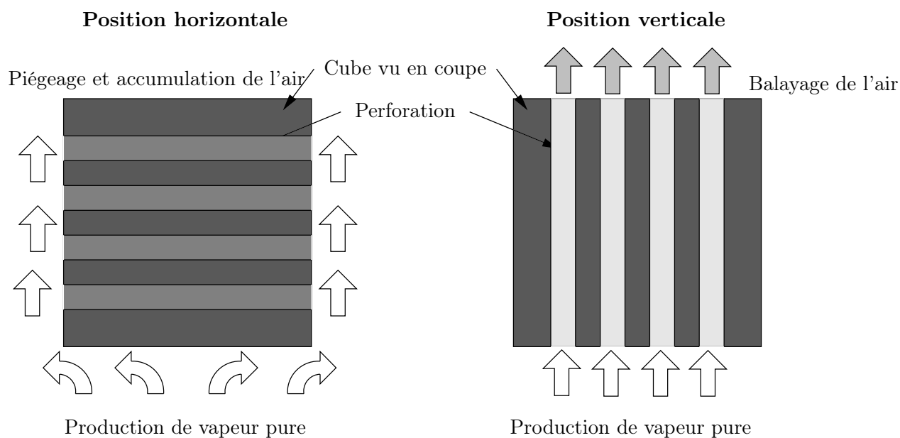
FIG. 5.47 – Description de l'influence de la géométrie de l'objet sur le balayage ou le piégeage de l'air
