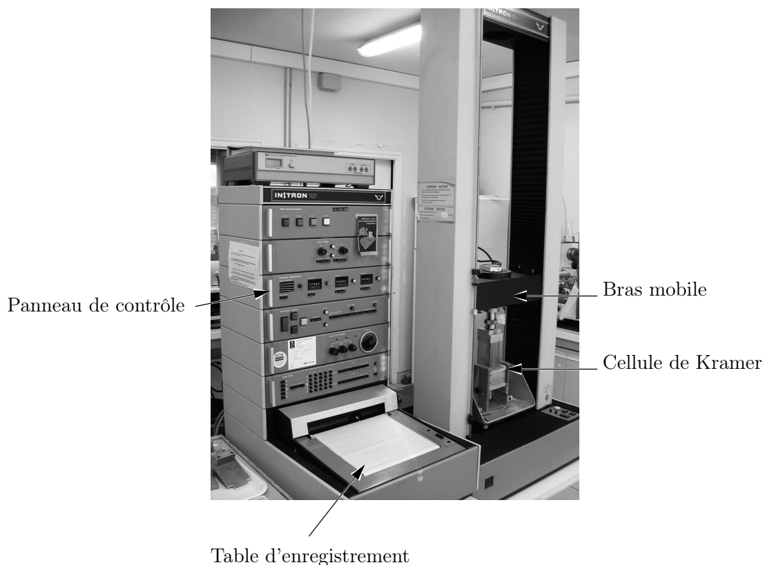
FIG. 3.26 – La machine d'essai bicolonne
