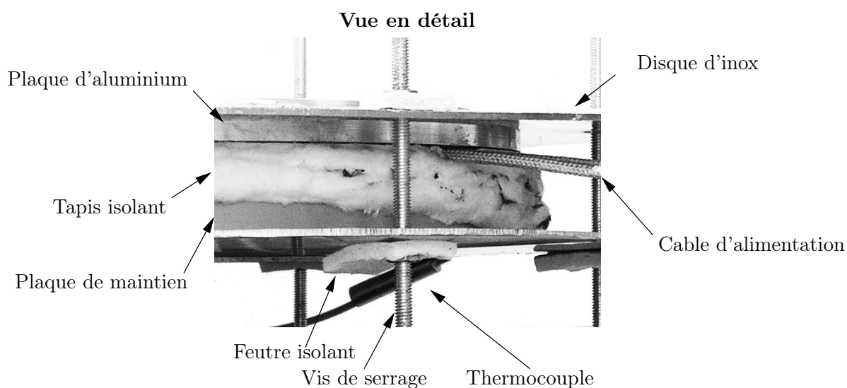
FIG. 7.2 – Description de la plaque de chauffe
