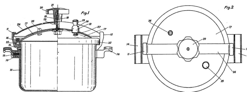
FIG. 1.1 – L'autocuiseur étrier
