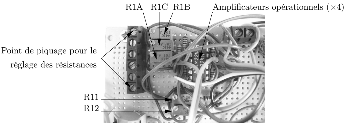
FIG. 7.8 – Localisation physique du réglage des commandes d'ouverture des vannes
