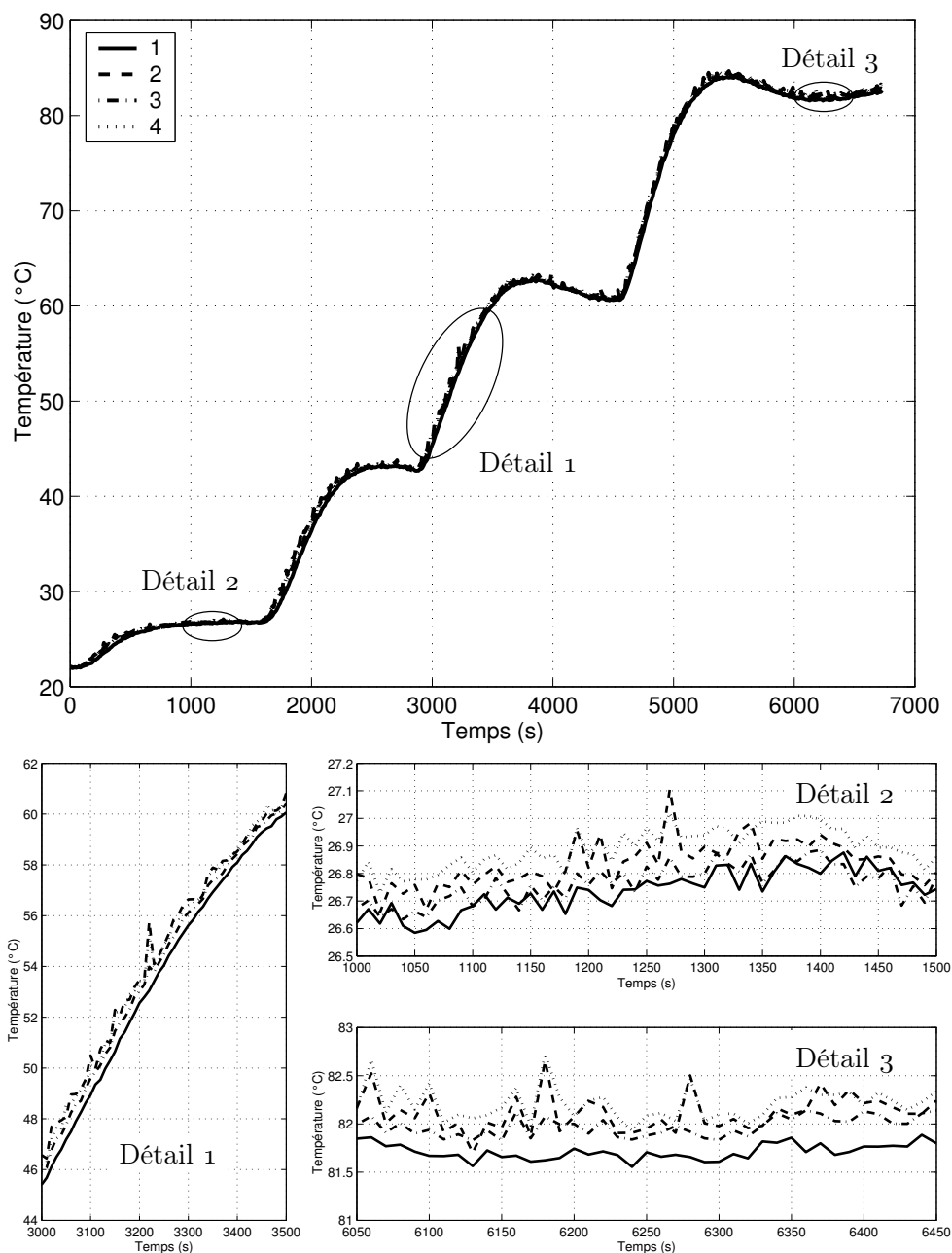
FIG. 3.7 – L'évolution de la température du mélange air-vapeur mesurée par différents thermocouples
